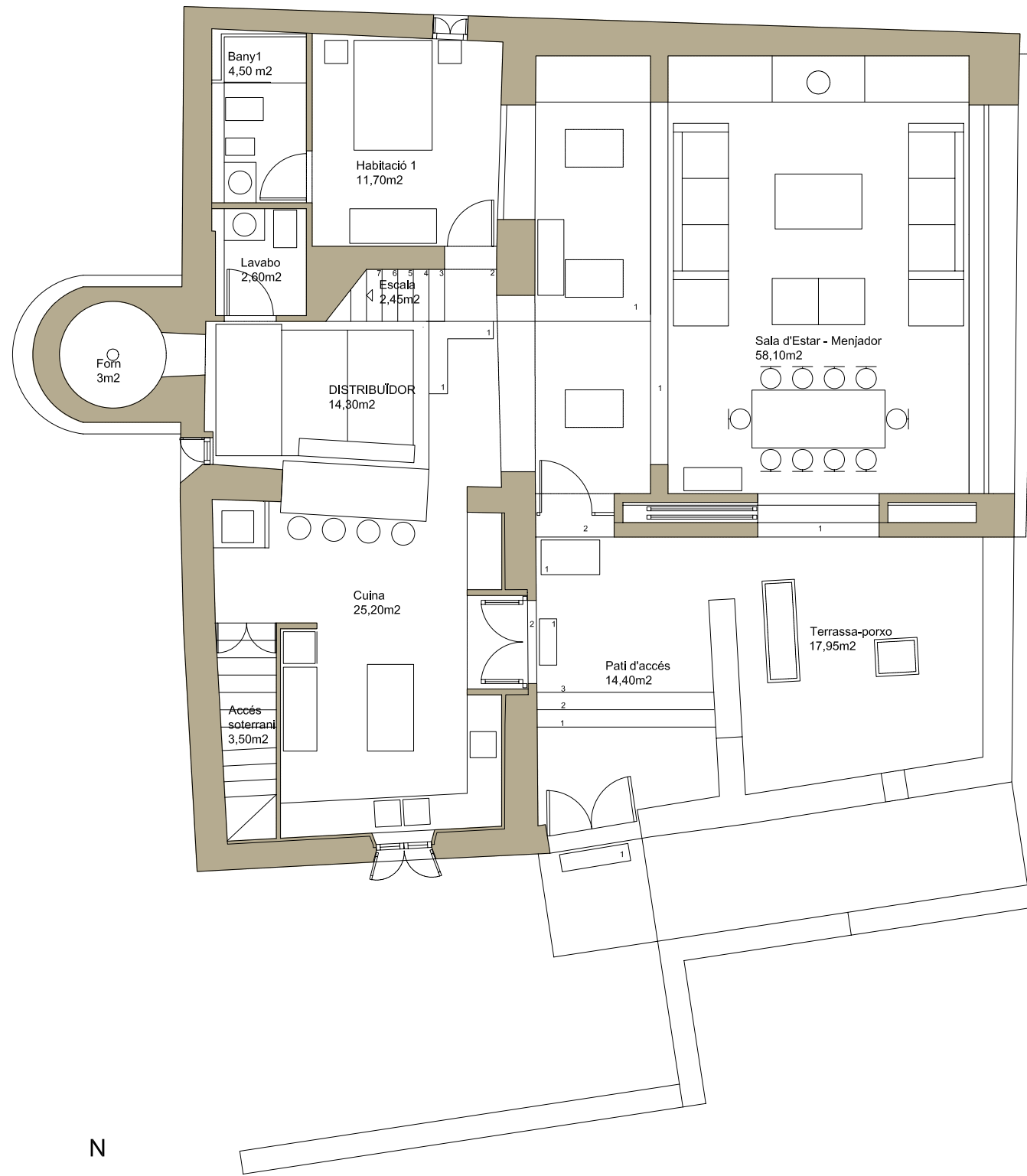
PLANTA BAIXA
